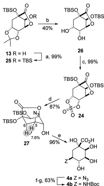
Scheme 11. Reagents and conditions: (a) TBSOTf, Py, DCM, 0 °C \rightarrow r.t.; (b) AcOH (aq., 80%), 65 °C; (c) (i) SOCl 2 , Et 3 N, DCM, r.t.; (ii) RuCl 3 ·3H 2 O (cat.), NaIO 4 , H 2 O, CCl 4 , CH 3 CN, r.t.; (d) (i) NaN 3 , DMF, 90 °C, (ii) H 2 SO 4 (70%), THF, r.t.; (e) (i) TFA (aq., 50%), 70 °C, (ii) LiOH, r.t., (iii) Amberlite IR-120 (H + ), r.t.; (f) Ac 2 O, Py, 0 °C \rightarrow r.t.; (g) H 2 , PtO 2 (cat.), Boc 2 O, THF, r.t.; (h) (i) LiOH, r.t., (ii) Amberlite IR-120 (H + ), r.t.
