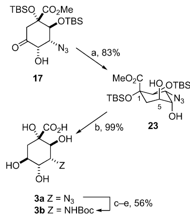
Scheme 9. Reagents and conditions: (a) NaBH 4 , MeOH, r.t.; (b) (i) TFA (aq., 50%), 70 °C, (ii) LiOH, r.t., (iii) Amberlite IR-120 (H + ), r.t.; (c) Ac 2 O, Py, 0 °C → r.t.; (d) H 2 , PtO 2 (cat.), Boc 2 O, THF, r.t.; (e) (i) LiOH, r.t., (ii) Amberlite IR-120 (H + ), r.t.
